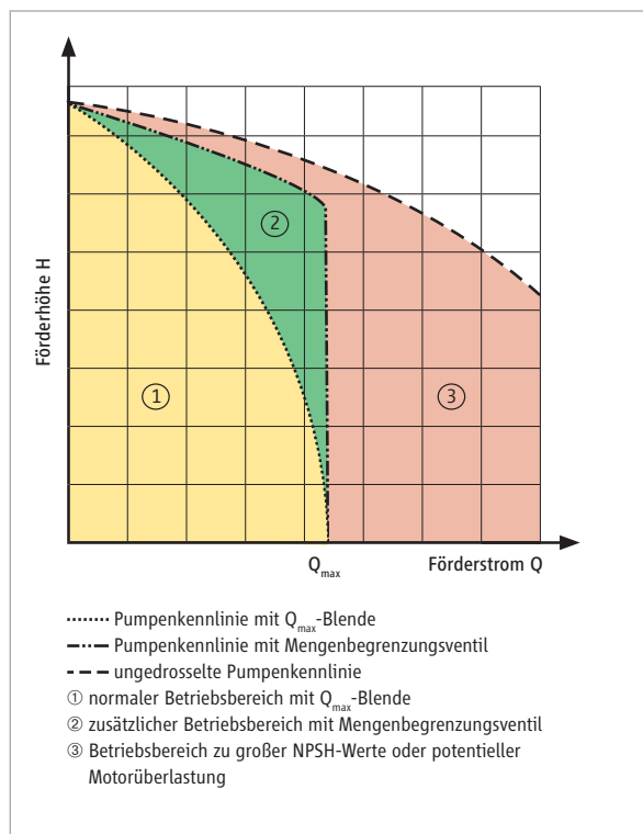
Abbildung 7: Pumpenkennlinien mit und ohne Q_{\max} -Absicherung
