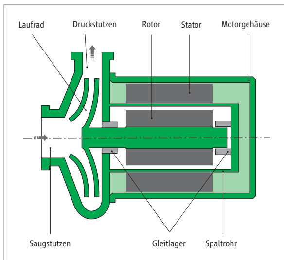
Abbildung 1: Schematische Darstellung einer Spalтроhrmotorpumpe
