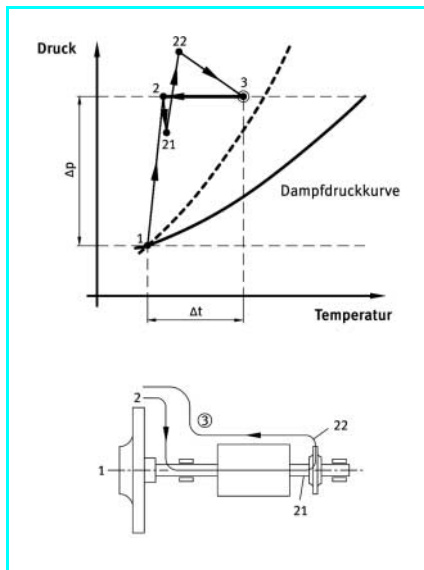
Bild 3: Druck-Temperatur-Diagramm bei Teilstromrückführung zur Druckseite
