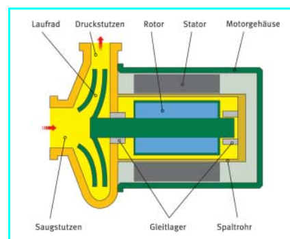
Bild 1: Schematische Darstellung einer Spaltrohrmotorpumpe
