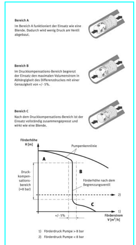
Bild 5: Funktionsschema des Mengenbegrenzungsventils
